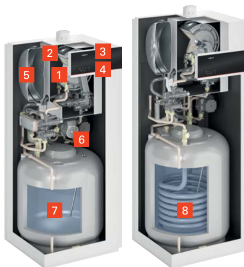
VITODENS 111-F (Tüüp B1TF)
